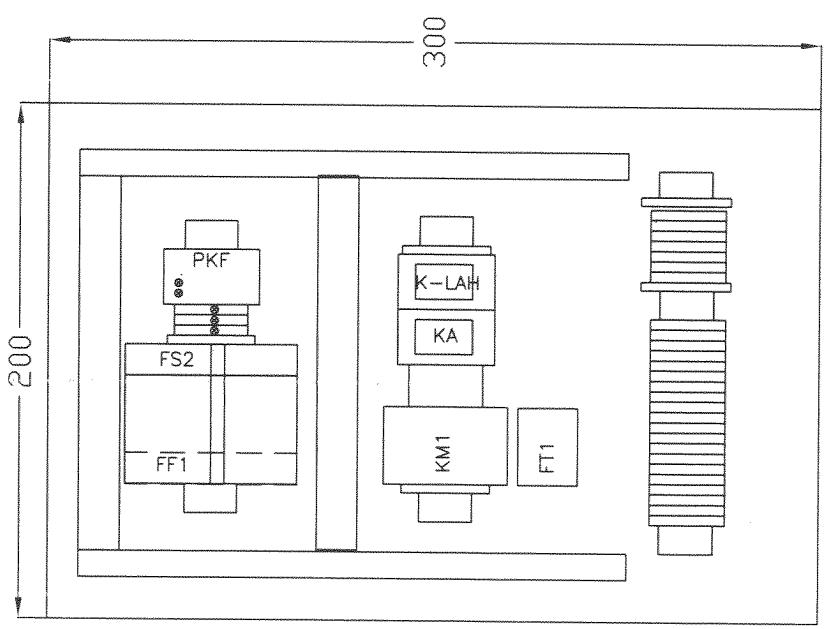
ELEWACJA SZAFKI
