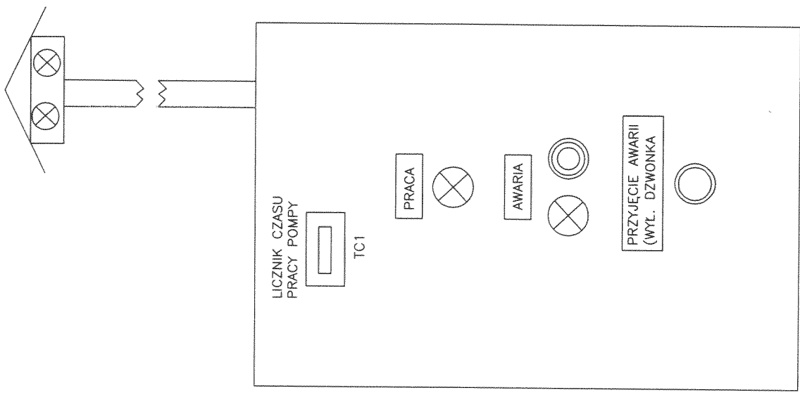
ELEWACJA SZAFKI
