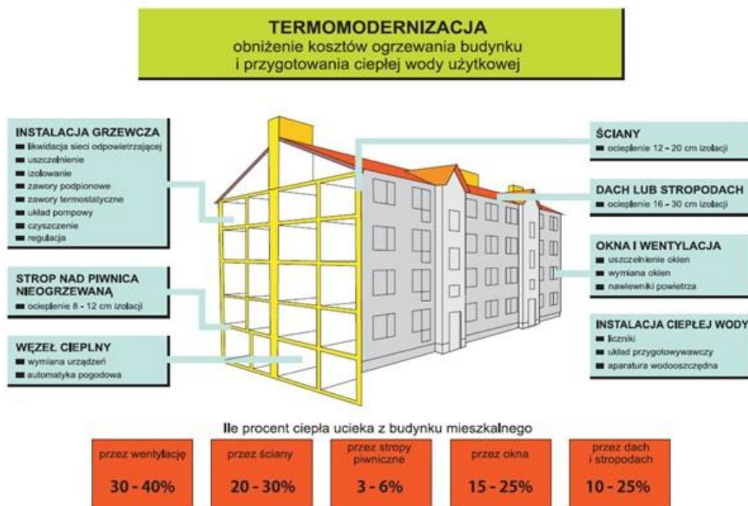
Ryc. 11. Termomodernizacja budynku
